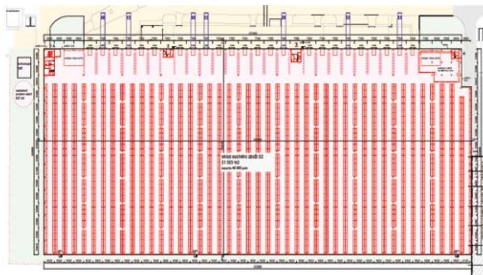
Půdorys nového suchého skladu S2
